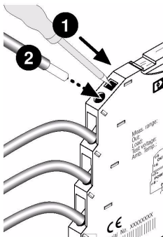
Figure 3 MINI MCR-SL-PT100-UI-SP MINI MCR-SL-PT100-UI-SP-NC
