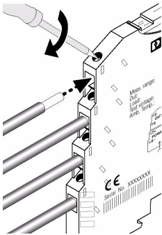
Figure 2 MINI MCR-SL-PT100-UI MINI MCR-SL-PT100-UI-NC
